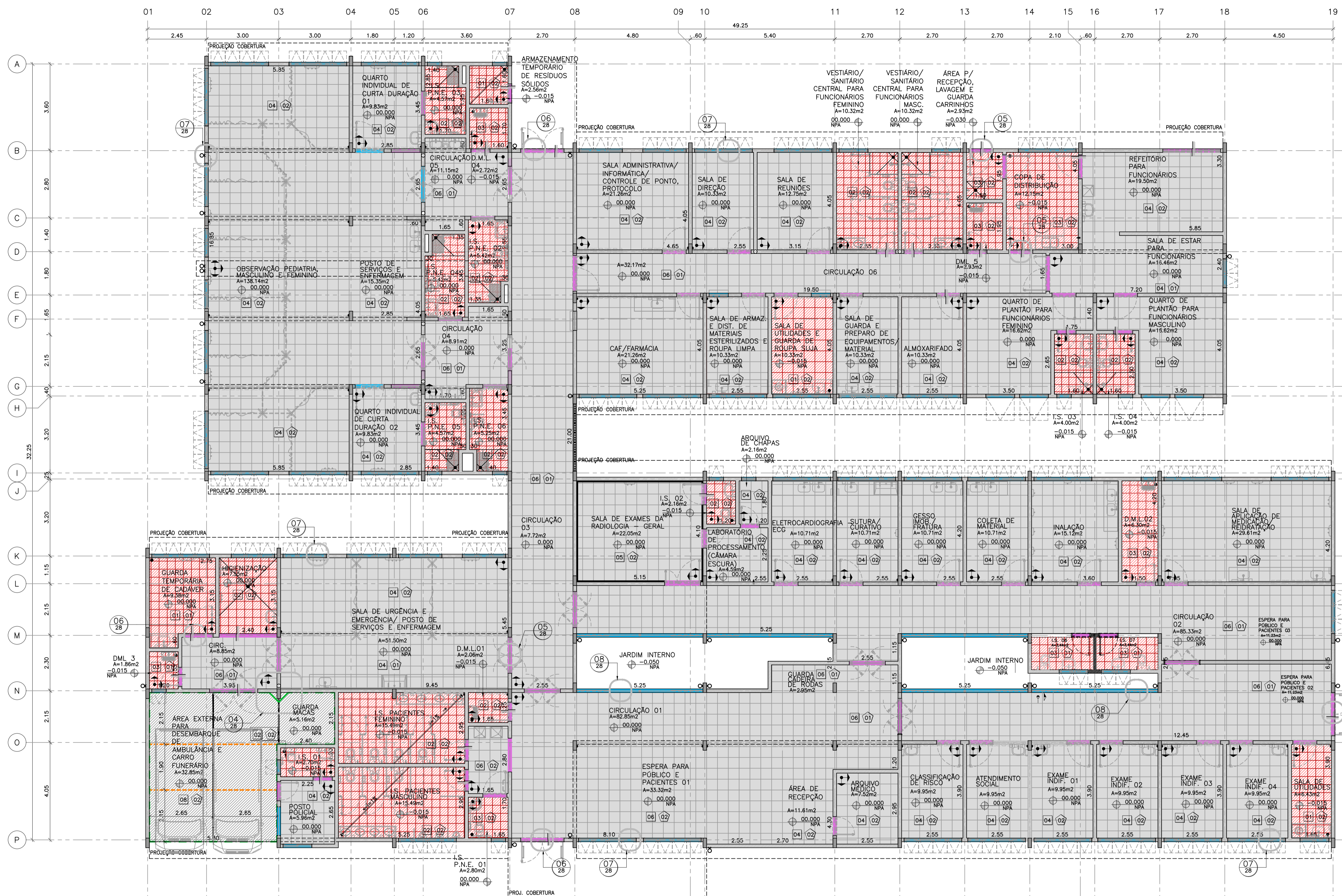
01 PAGINAÇÃO E DETALHAMENTO DE PISOS PLANTA TERREIA ESCALA: 1:75
